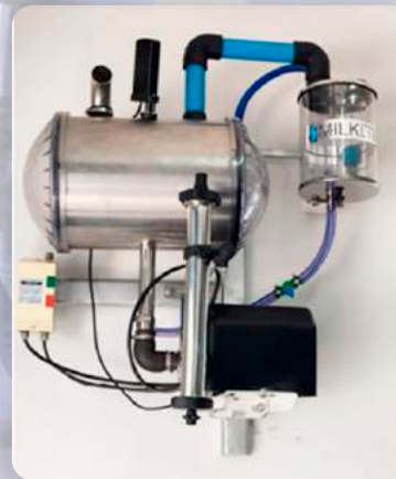
EQUIP. DE ORD. UNID. FINAL 40 LTS GARRAÇÃO HORIZONTAL Cód. 14106
